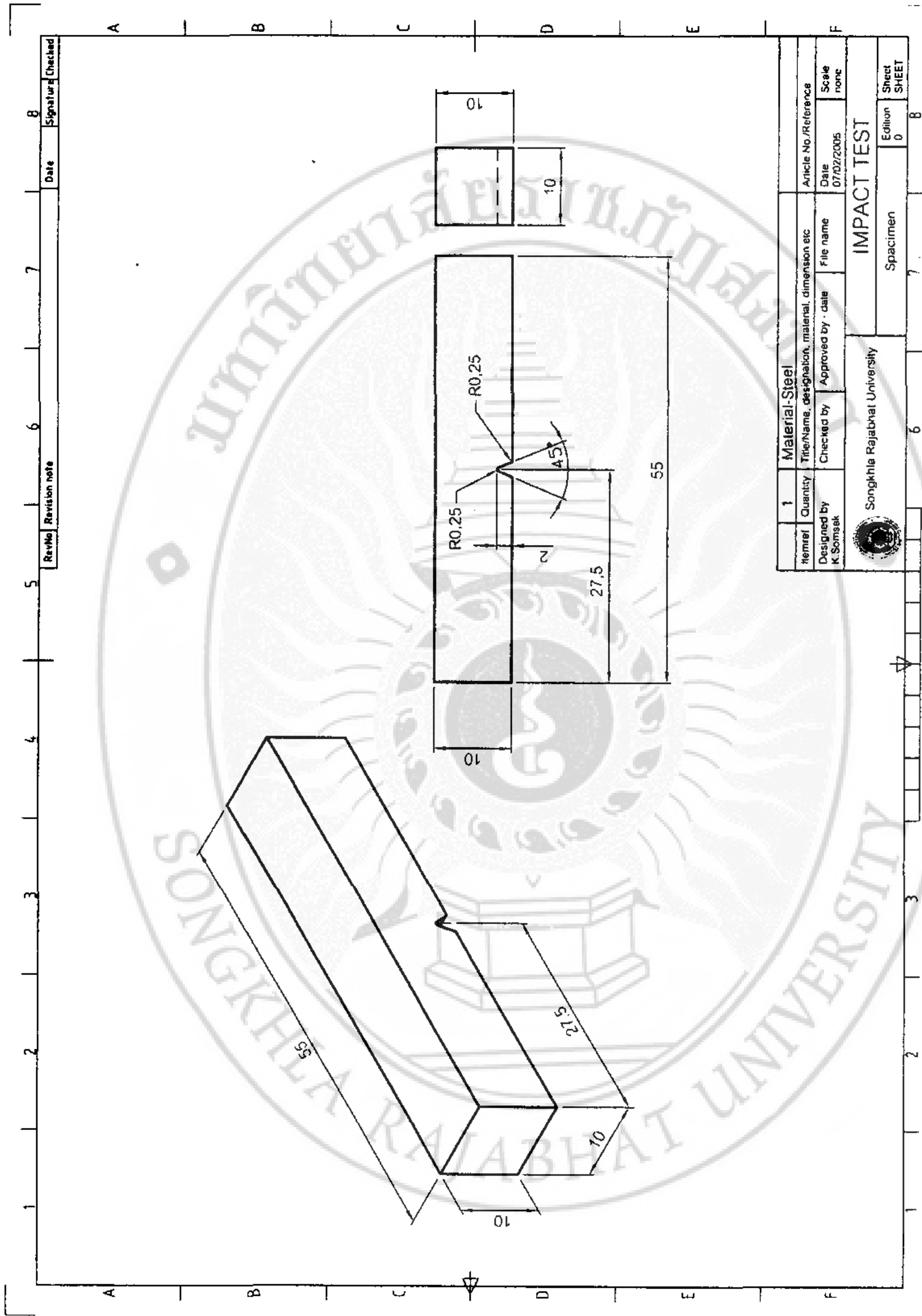
รูปที่ ข.2 Drawing ของชิ้นทดสอบแรงกระแทก
