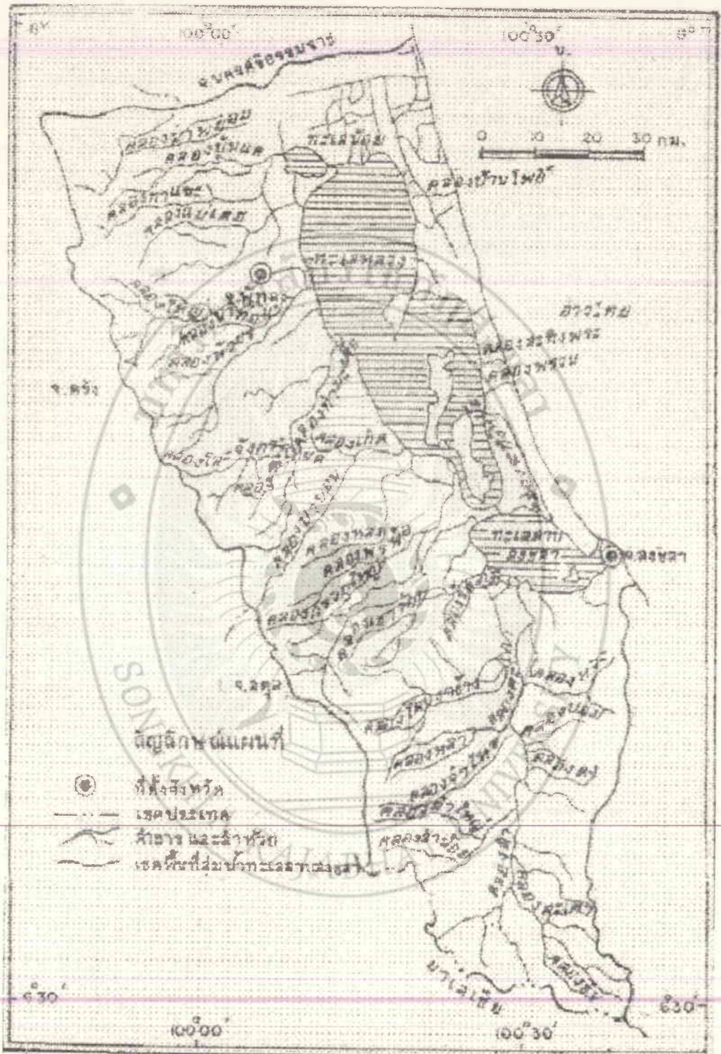
ภาพที่ 2.2: ระบบลำน้ำของกลุ่มน้ำทะเลสาบสงขลาโดยสังเขป
